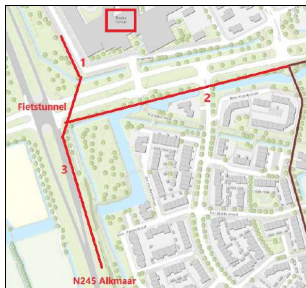
Afb. 16 Fietstunnel van 1 naar 3
